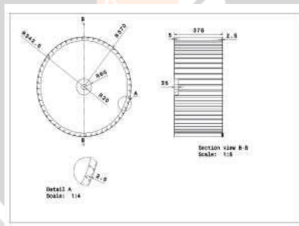
Fig. Drafting of Blower Fan
