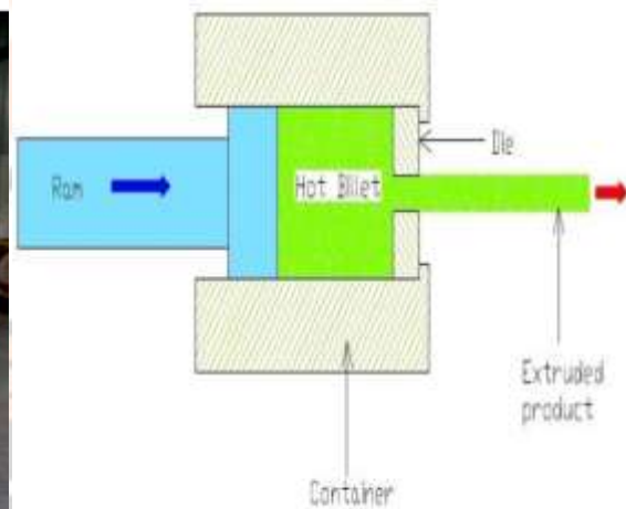
Fig.3.2 Extrusion die
