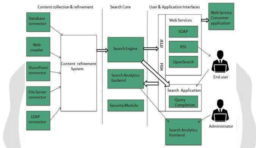
Fig. 1: Keyword
