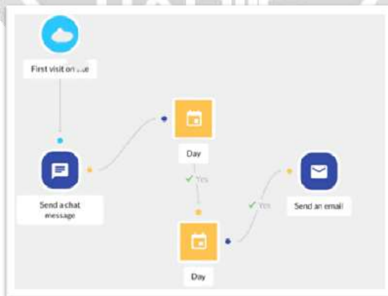
Fig. 2: Chat API
